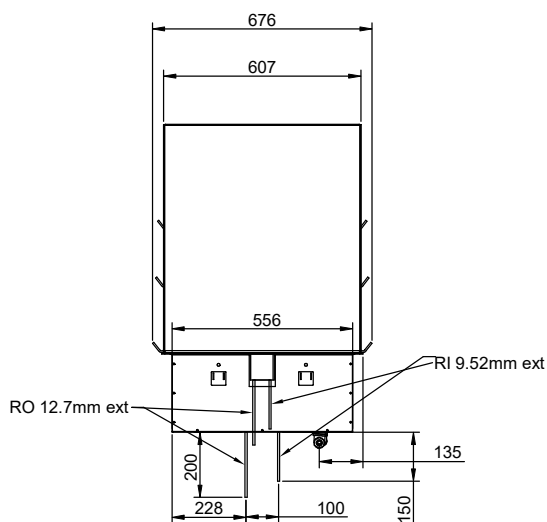
Boční
